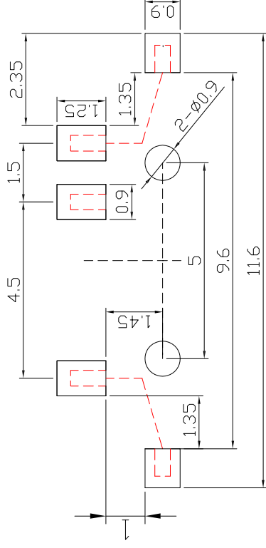
安装图 (PCB LAYOUT PLAN)
